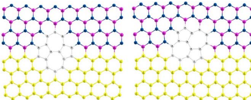
Рис. 2. Оптимизированные GBNC (C 68 B 34 N 34 H 32 ) с дефектами Стоуна-Уэльса, образующимися при повороте “прямой” 1 (слева) и “наклонной” 2 (справа) связей (см. рис. 1). Дефекты Стоуна-Уэльса помечены серым цветом.
