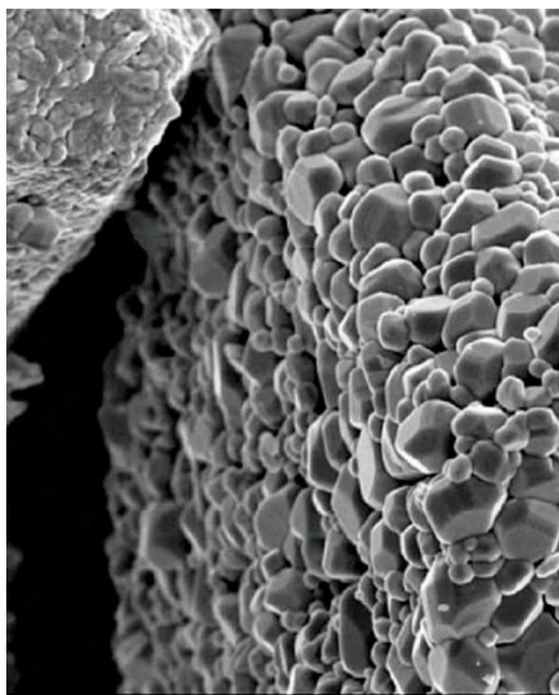
«Странный оксид вольфрама». Продукт термического разложения солей изополивольфраматовых кислот. Формирование сложной структурной организации кристаллитов оксида вольфрама (VI), полученных в результате термического разложения солей изополивольфраматовых кислот
