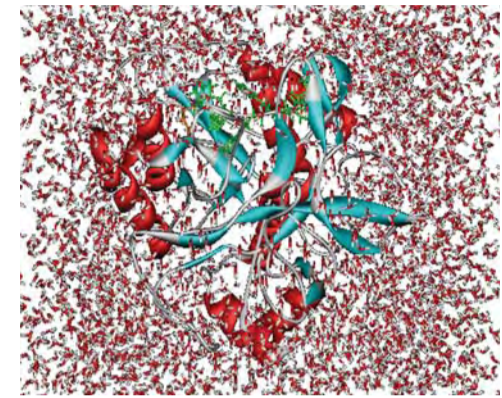
Пример структуры гидратированного фермента. Сольватная оболочка белка построена методами молекулярной механики
