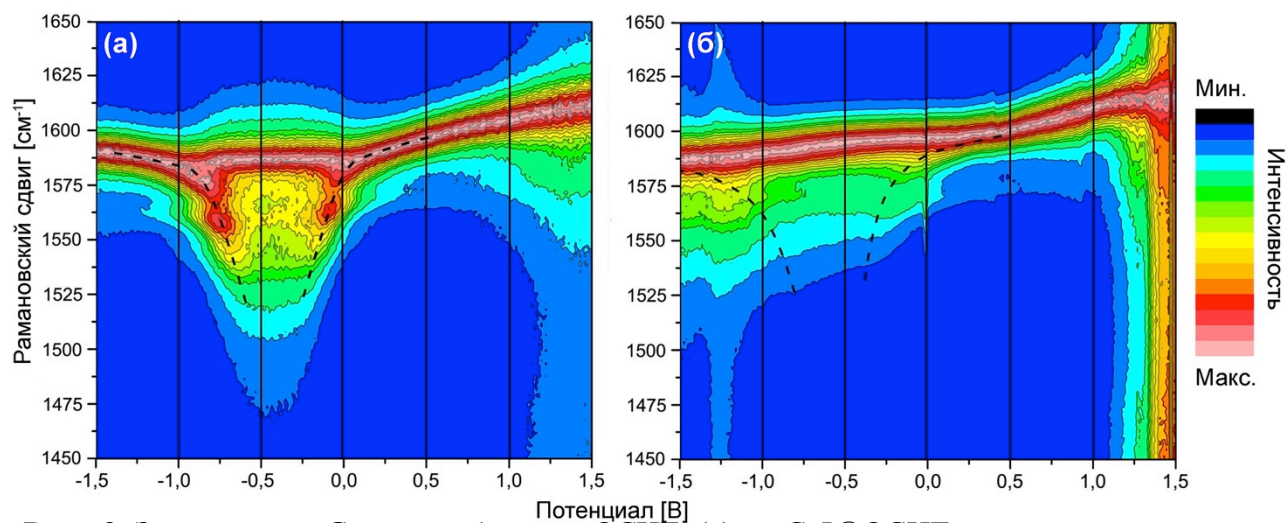
Рис. 3 Зависимость G-моды образцов ОСНТ (а) и CuI@ОСНТ при электрохимическом зарядении.
