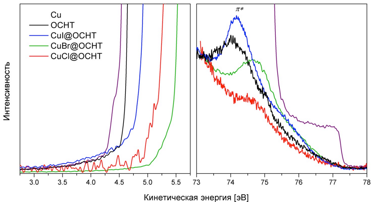
Рис. 4 Фотоэлектронный спектр вторичных электронов (а) и валентной зоны (б) незаполненных ОСНТ, нанокompозитов CuX@ОСНТ и Cu, полученные при энергии излучения h\nu = 77.3 эВ
