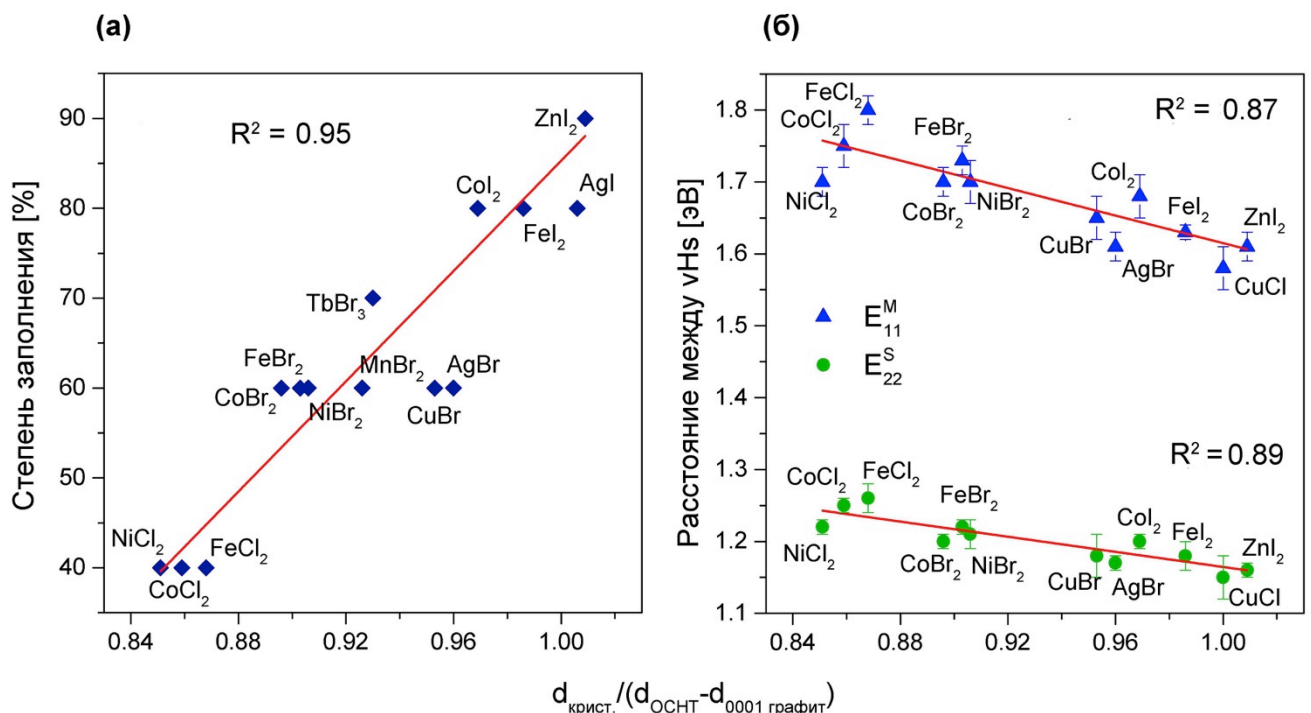
Рис. 4.23 Зависимость степени заполнения ОСНТ (а), а также расстояния между сингулярностями ван Хова (б) от соотношения диаметра внедренного кристалла и ОСНТ.
