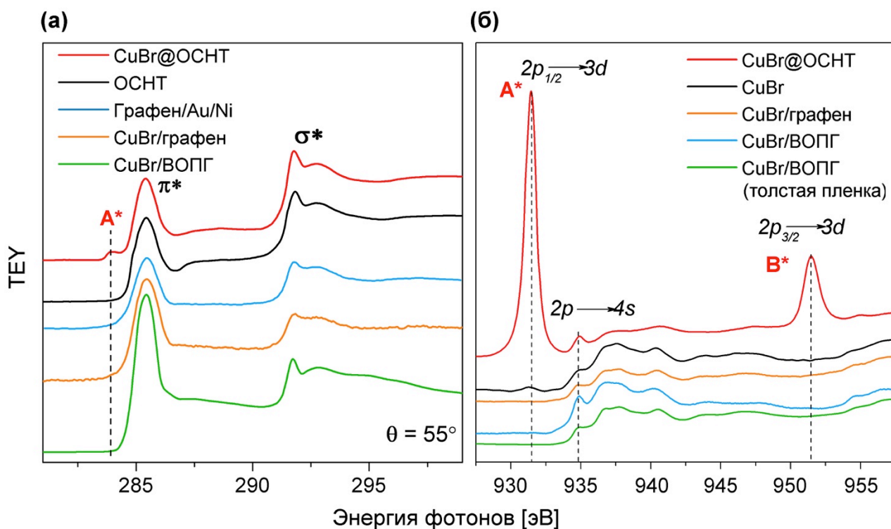
Рис. 7 Спектры рентгеновского поглощения СК-края (а) и CuL_{2,3} -края (б) исходных и допированных CuBr ОСНТ, графена и графита.
