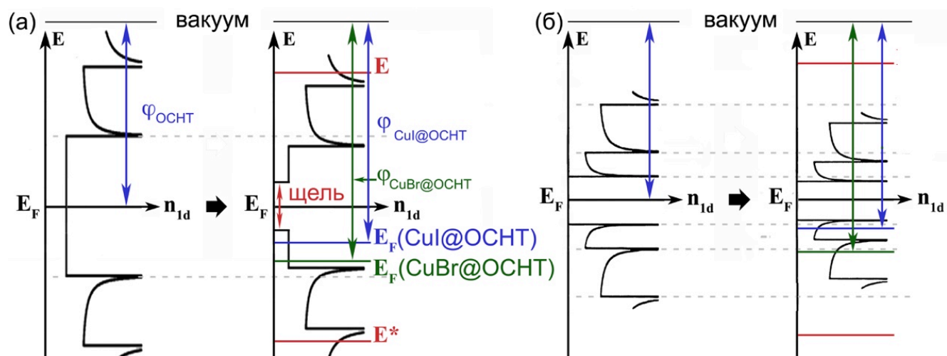
Рис. 5 Изменение электронной структуры металлических (а) и полупроводниковых (б) ОСНТ в результате интеркаляции \text{CuHal@ОСНТ} . Красным отмечен новый уровень
