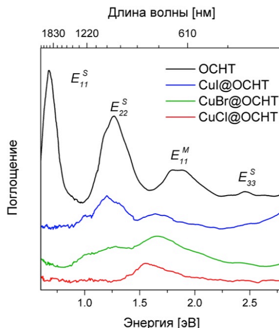
Рис. 2 Спектры оптического поглощения незаполненных ОСНТ и нанокомпозитов CuX@ОСНТ.
