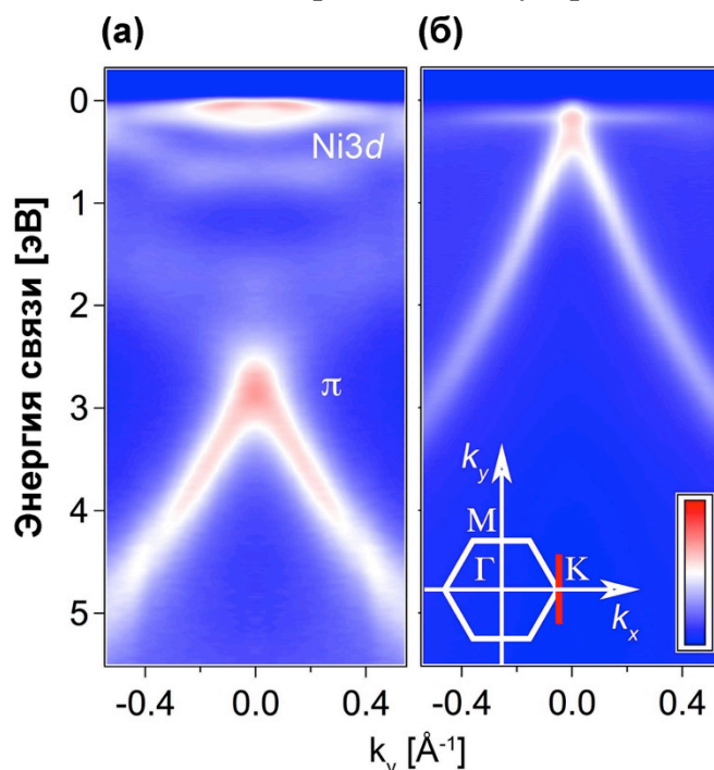
Рис. 8 Данные ФЭСУР графена на подложке Ni(111) до (слева) и после (справа) интеркаляции Ge.
