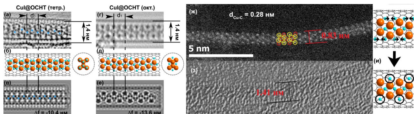
Рис.1 Микрофотографии (а, г), расчетные модели структуры (б, д) и моделированные ПЭМ изображения (в, е) на их основе для CuI@ОСНТ . HAADF (ж) и STEM (з) данные CuI@ОСНТ . Атомы Cu отмечены желтым, а I красным. Изменение структуры одномерного кристалла (в).
