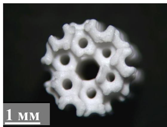
Рис. 13. Фотография керамического каркаса цилиндрической формы со структурой Кельвина вдоль направления [111]. Диаметр пор 500 мкм.
