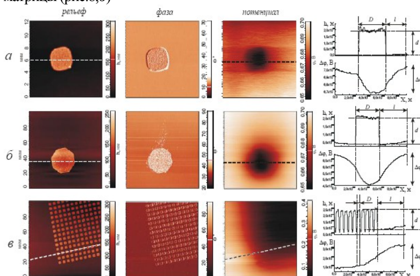
Рис.8. Двумерные АСМ изображения рельефа (колонка “рельеф”), фазы (колонка “фаза”) и КРП (колонка “потенциал”) поверхности nGaAs(100) с концентрацией носителей заряда N_D=6 \cdot 10^{16} \text{ см}^{-3} с расположенными на ней диодными матрицами (в), образованными металлом платина (Pt) с диаметром 5 мкм и толщинами 0,2 мкм (а) и 0,1 мкм (б) с соответствующими профилями продольных сечений пространственного h(x) и потенциального \Delta\varphi(x) рельефов.
