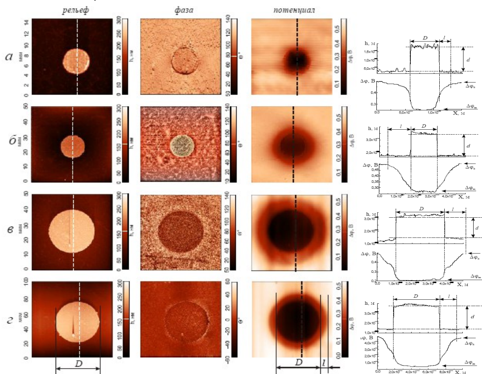
Рис. 2. Двумерные АСМ изображения рельефа, фазового контраста, КРП, пространственных h(x) и потенциальных \Delta\phi(x) сечений рельефов поверхности nGaAs(100) с концентрацией доноров 3 \cdot 10^{15} \text{ cm}^{-3} с расположенными на ней металлом (Au) толщиной d \approx 0,2 \text{ мкм} с диаметрами D: а) 5 мкм; б) 15 мкм; в) 30 мкм и г) 50 мкм.
