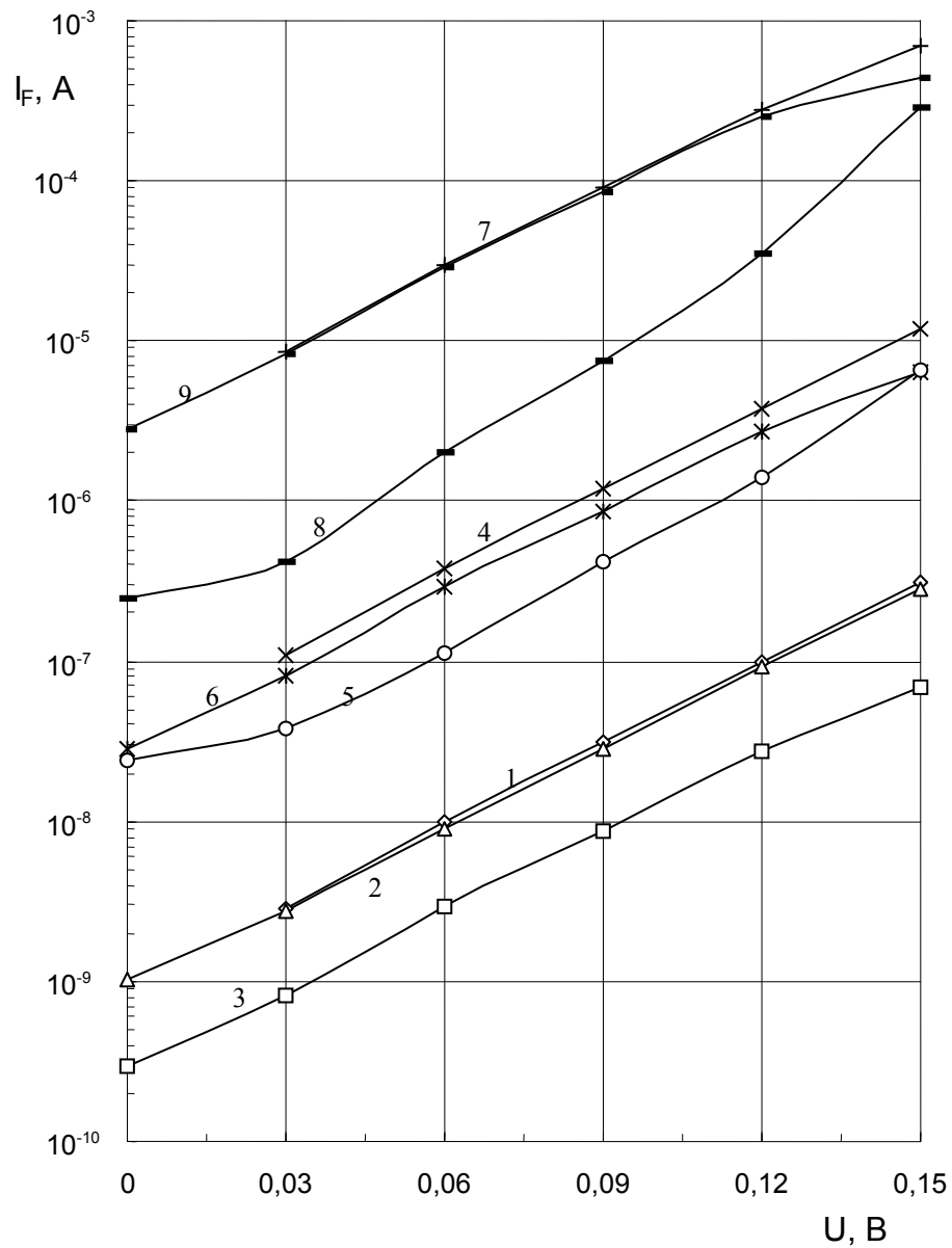
Рис.11. Прямые ветви ВАХ Cr - nSi диодов Шоттки с диаметрами 10 мкм, 100 мкм и 1000 мкм: токи общего контакта I_F (кривые 1, 4 и 7, соответственно), периферийные токи I_{LS} (кривые 2, 5 и 8, соответственно), токи общего контакта без влияния периферийных эффектов I_S (кривые 3, 6 и 9, соответственно).
