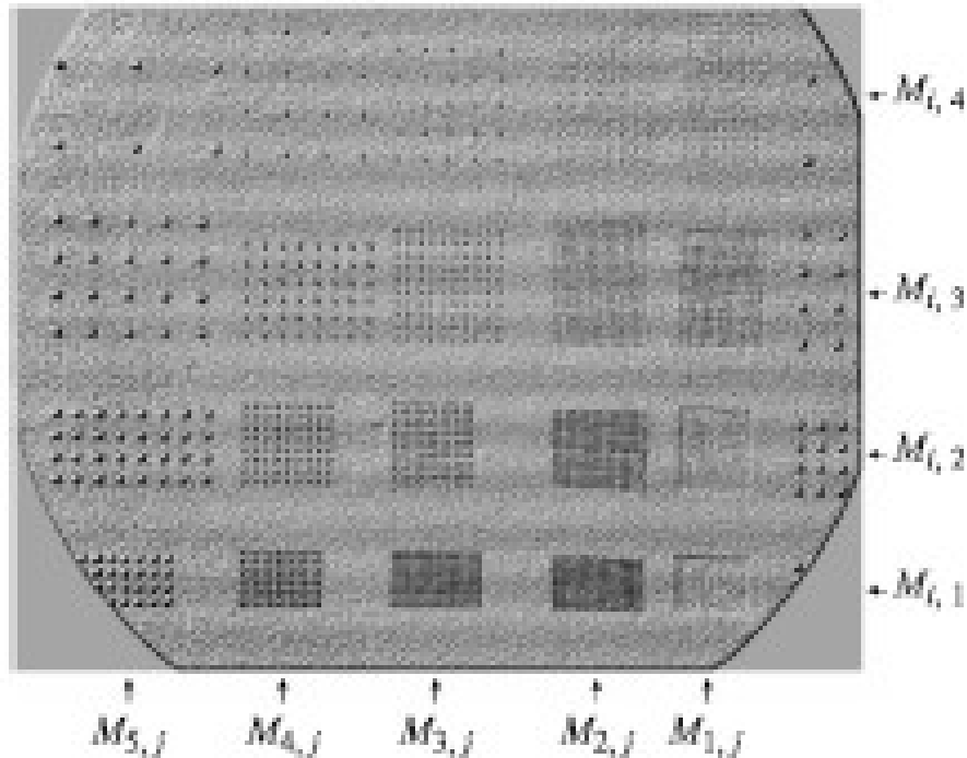
Рис.15. Фотография поверхности чипа эпитаксиального pGaAs с расположенными на ней матрицами M_{i,j} (где, D_{i,j} - диаметр контактов, H_{i,j} - расстояние между контактами) золотых контактов ДШ. Целое число “i” нумерует диаметр контактов: 1 – D_{1,j} = 3 , 2 – D_{2,j} = 5 , 3 – D_{3,j} = 10 , 4 – D_{4,j} = 15 и 5 – D_{5,j} = 30 мкм. Целое число “j” нумерует расстояние между контактами: 1 – H_{i,1} = 1 \times D_{i,1} , 2 – H_{i,2} = 2 \times D_{i,2} , 3 – H_{i,3} = 4 \times D_{i,3} и 4 – H_{i,4} = 10 \times D_{i,4} .
