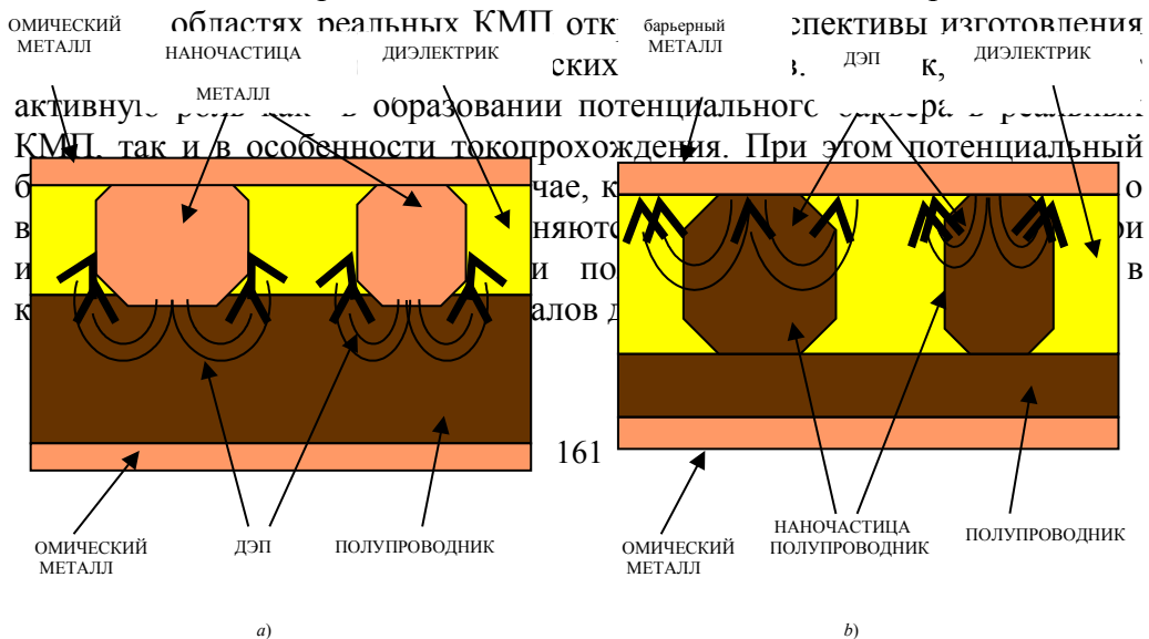
Рис.23. Принципиальные структуры nano - КМП с ДЭП полупроводниковых преобразователей на основе металлических (a) и полупроводниковых (b) наночастиц.
