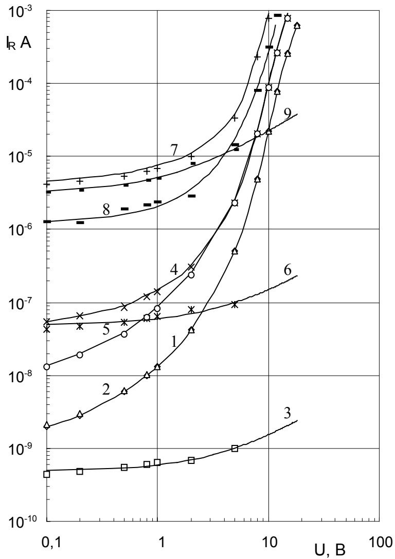
Рис.12. Обратные ветви ВАХ Cr - nSi диодов Шоттки с диаметрами 10 мкм, 100 мкм и 1000 мкм: токи общего контакта I_F (кривые 1,4 и 7, соответственно), периферийные токи I_{LS} (кривые 2,5 и 8, соответственно), токи общего контакта без влияния периферийных эффектов I_S (кривые 3, 6 и 9, соответственно).
