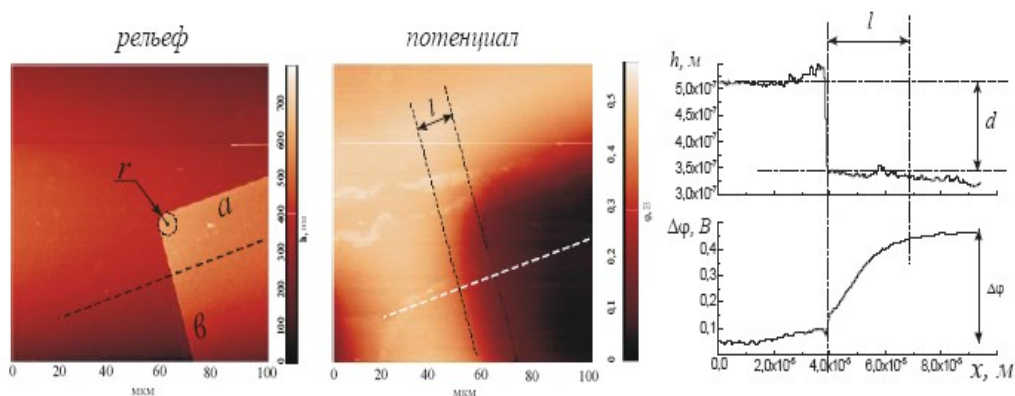
Рис.4. Двумерные АСМ изображения рельефа (колонка “рельеф”), КРП (колонка “потенциал”) поверхности эпитаксиального pGaAs(100) с концентрацией носителей заряда N_D = 3.10^{15} \text{ см}^{-3} с расположенными на ней прямоугольным 100 \times 300 \text{ мкм}^2 Au-контактом толщиной 0,17 \text{ мкм} и соответствующими профилями продольных сечений пространственного h(x) и потенциального \Delta\varphi(x) рельефов по пунктирным линиям.
