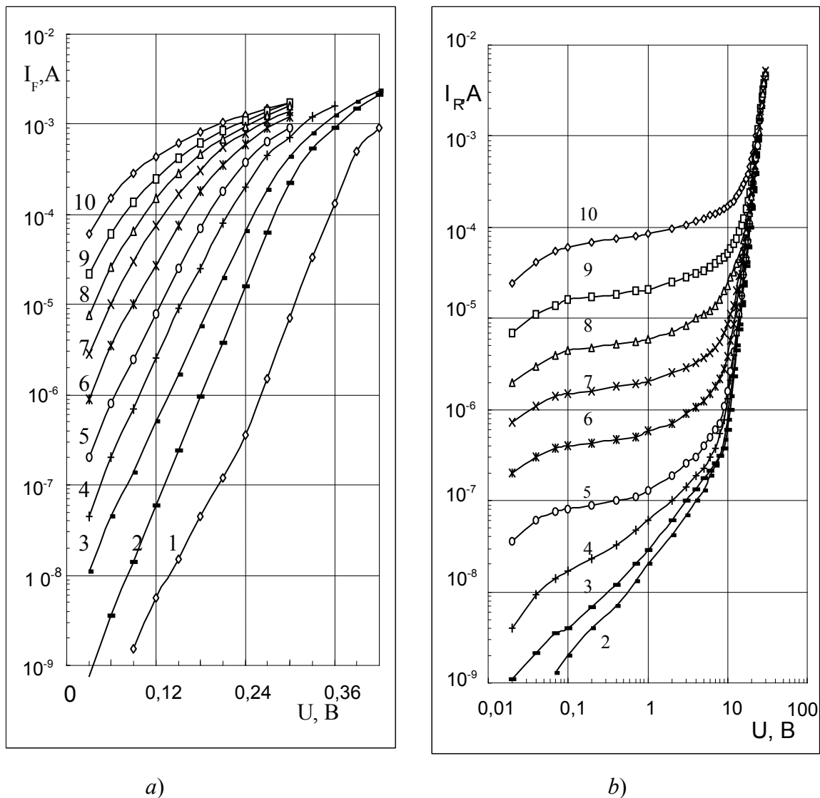
Рис.13. Прямые (a) и обратные (b) ветви ВАХ Ni - nSi диодов Шоттки с диаметром 100 мкм при температурах T (K): 1 – 185, 2 – 222, 3 – 247, 4 – 267, 5 – 292, 6 – 311, 7 – 329, 8 – 345, 9 – 363, 10 – 387.
