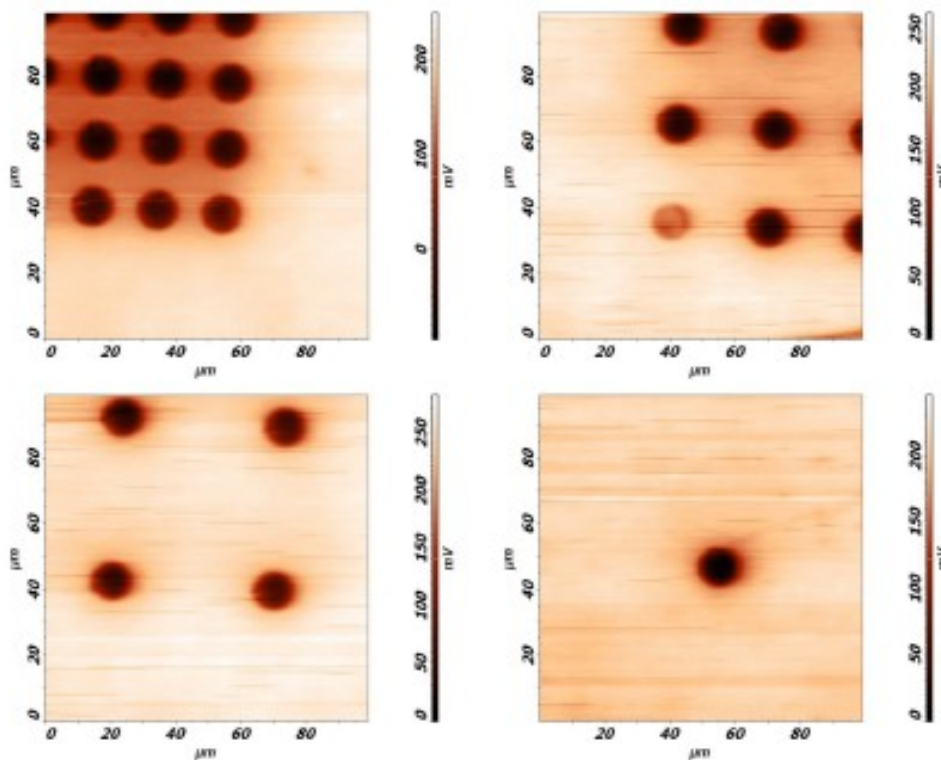
Рис. 6. АСМ изображения КРП эпитаксиального Au - nGaAs(100) контактов с диаметром 10 мкм и толщиной металла 0,060 мкм при разной кратности расстояний между ними.
