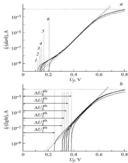
Рис.19. Прямые ветви вольтамперных характеристик Au-pGaAs ДШ одинаковой площадью S_i = 7853,98 \text{ мкм}^2 разными ( i ) формами (см.рис.19). a – темновые (dark) и b – световые (light)
