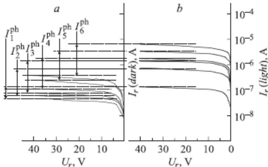
Рис.20. Обратные ветви вольтамперных характеристик Au-pGaAs ДШ одинаковой площадью S_i = 7853,98 \text{ мкм}^2 разными ( i ) формами (см.рис.18). a – темновые (dark) и b – световые (light)
