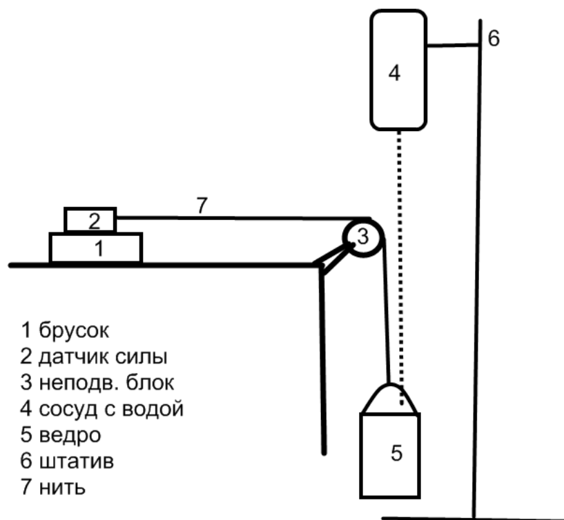
Схема экспериментальной установки
