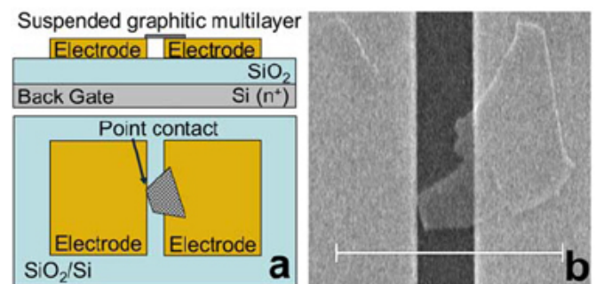
Рис. 1. Схема структуры с точечным контактом из графена (а) и вид сверху реальной структуры (b).
