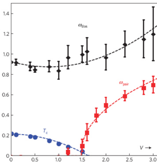
Фазовая диаграмма разупорядоченного s -волнового сверхпроводника в координатах температура (вертикальная ось) – сила беспорядка V .
