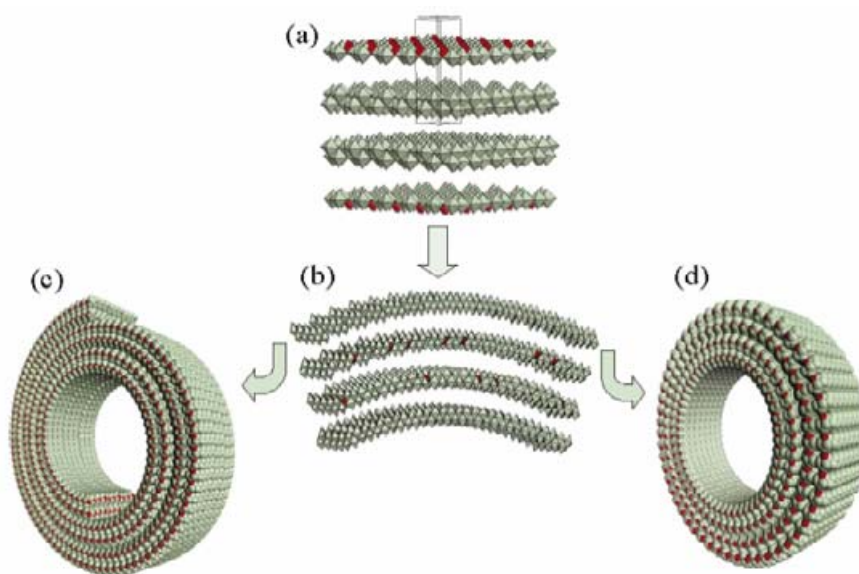
Нанотубулярная форма V_2O_5 после гидротермальной обработки с поверхностно-активным веществом.
